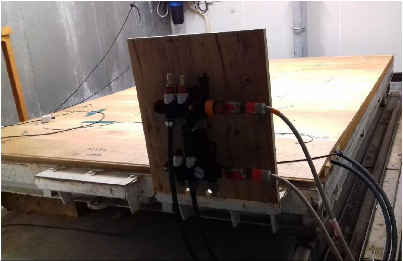
Maquette d'essai du Système Parquet sur sol chauffant rafraichissant 3mx2m avec systèmes de capteurs de mesure température et humidité
