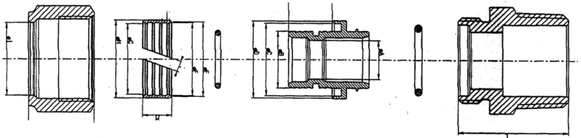
Figure 1 - Raccord GIACO - Schéma de principe
