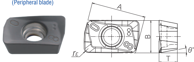
Fig.5(外周刃) (Peripheral blade)
