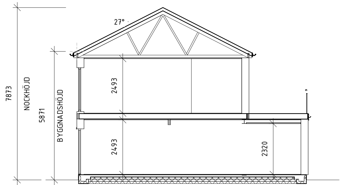
SKÅNETAKFOT SEKTION B-B
