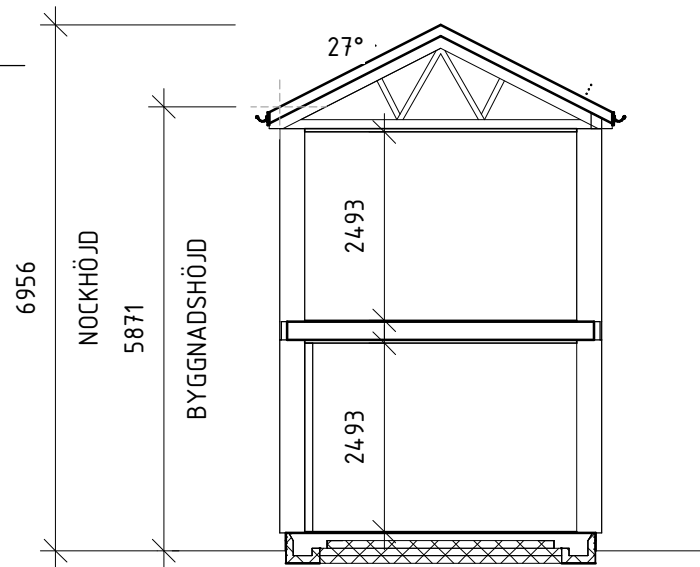
SKÅNETAKFOT SEKTION C-C
