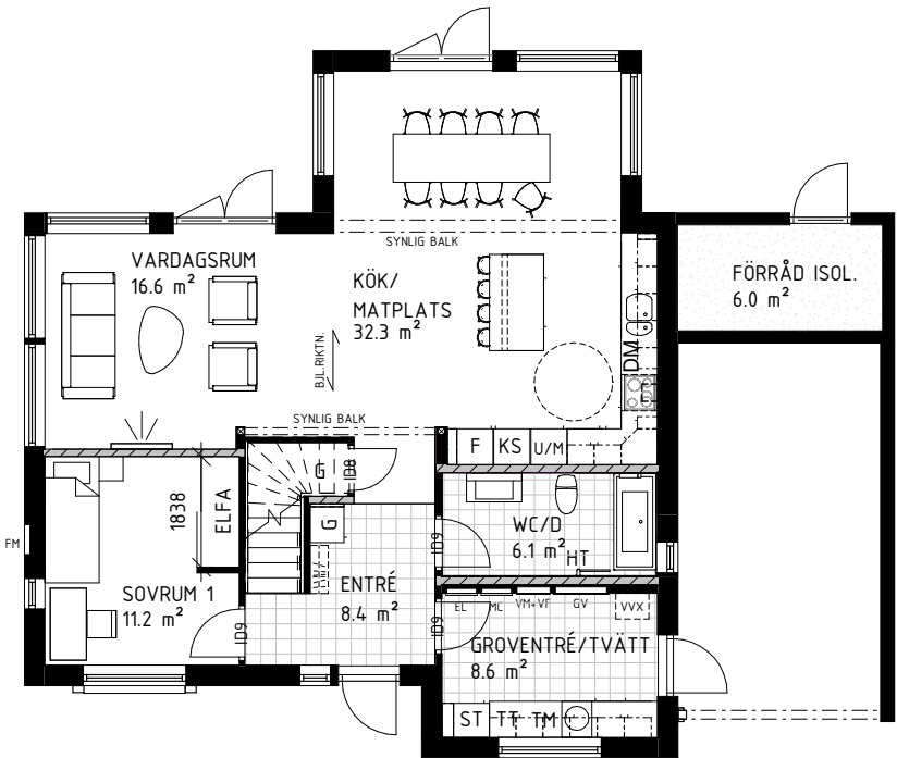
Hus C och D Alternativ planlösning, plan 1 Inbyggd trappa Planlösning visar även tillval Elfa och överskåp i Groventré/Tvätt.
