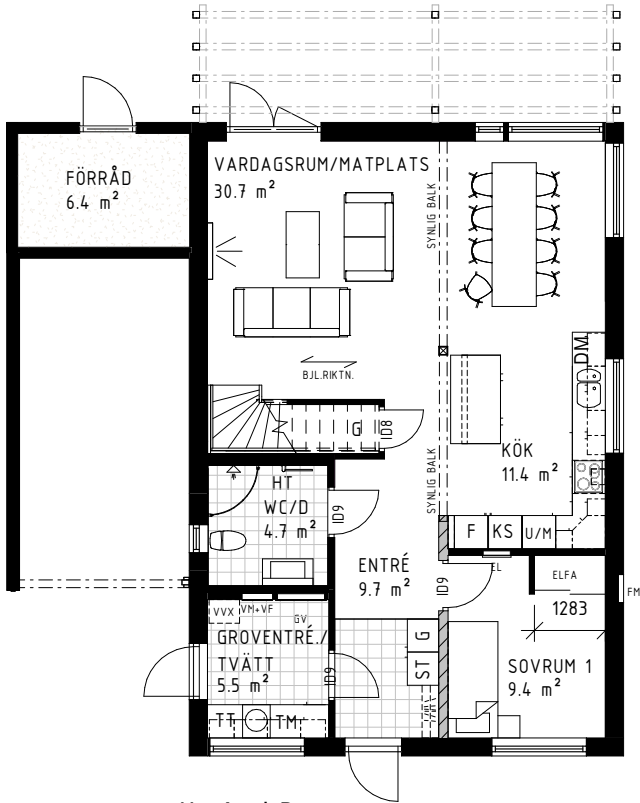
Hus A och B Alternativ planlösning, plan 1 Inbyggd trappa
