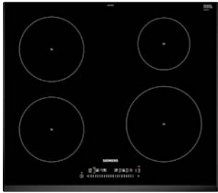
Induktionshäll EH651FEB1E • PowerBoost-funktion för alla induktionszoner • TouchSlider-styrning • 17 effektlägen • Timer med avstängningsfunktion per kokzon
