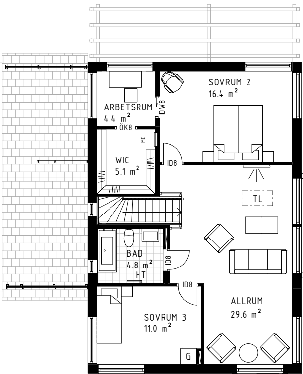
Hus A och B Alternativ planlösning, plan 2 Stort allrum istället för Sovrum 4
