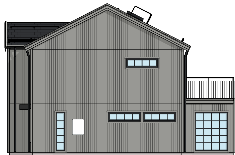
FASAD HÖGERSIDA
